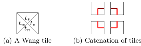
Fig. 2. Wang tiles
